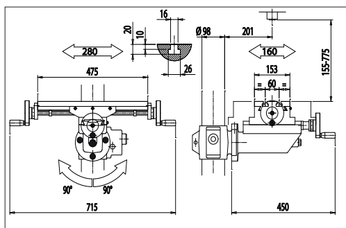
TC: Tavola Croce per serie V.
