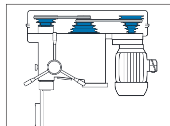
PU: Pulegge a gradini V30
