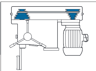
PU: Pulegge a gradini V22 - V22E
