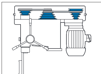
PU: Pulegge a gradini V25 - V25E.
